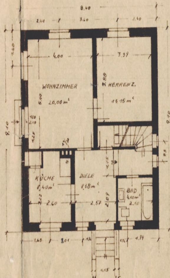
ERDGESCHOSS
