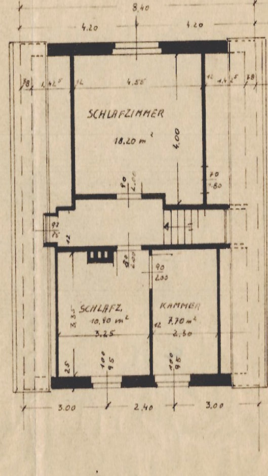
DACHGESCHOSS
