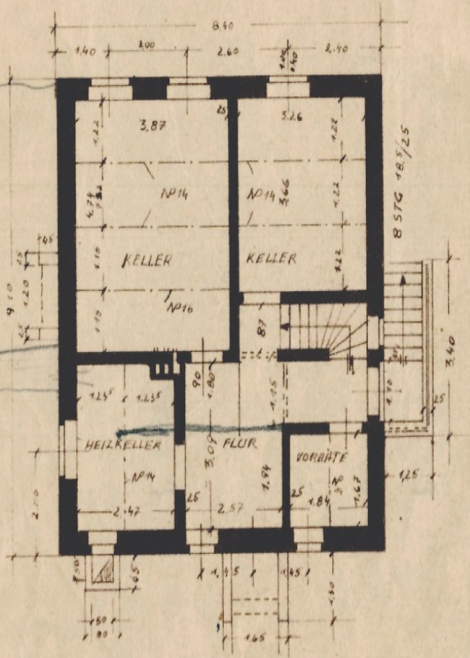
KELLERGESSCHOSS
